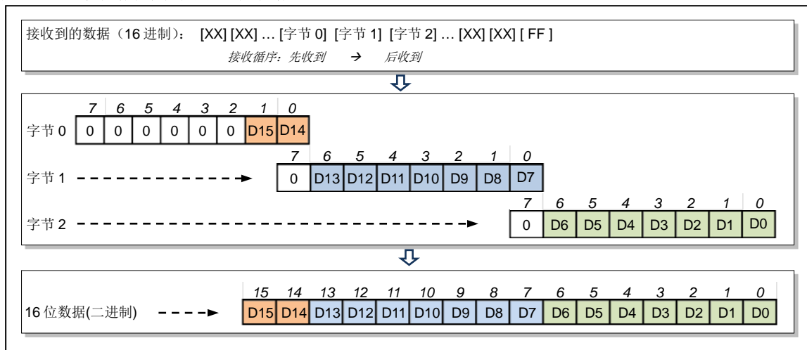
图 12-1: 3 个数据字节转化为 16 位数据
