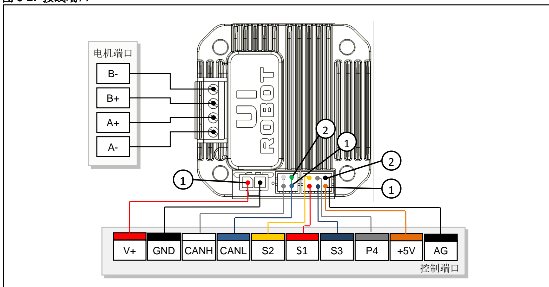
图 0-2: 接线端口
