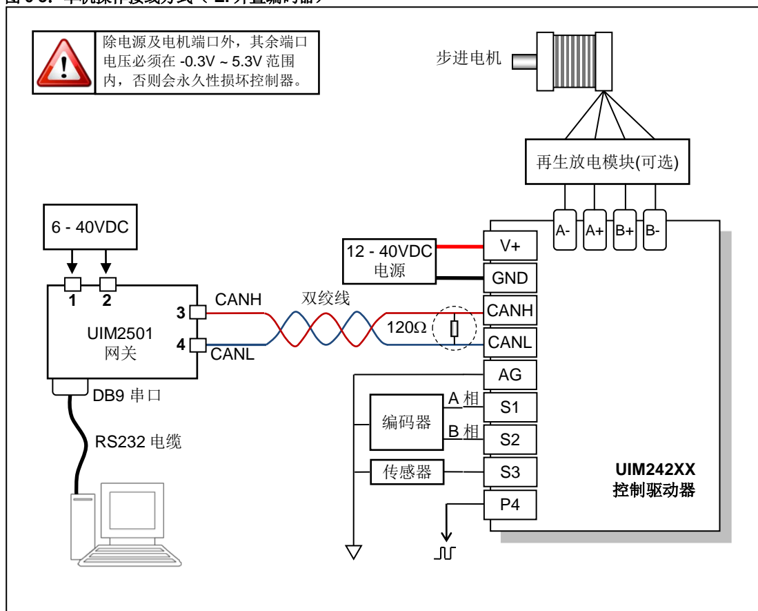
图 0-3: 单机操作接线方式 (-E: 外置编码器)
