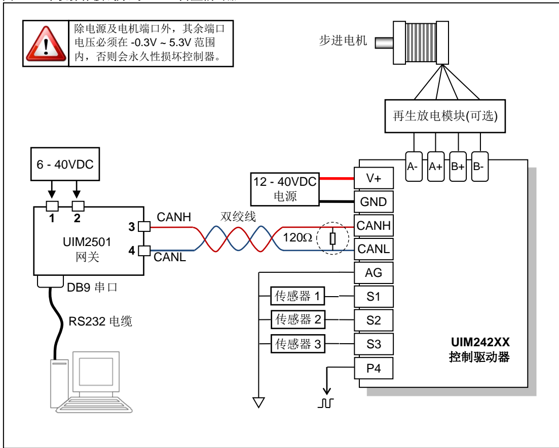
图 0-4：单机操作接线方式（-IE：内置编码器）
