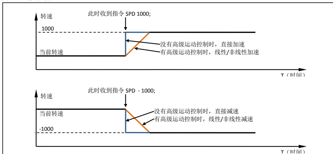
图 6-1 速度控制
