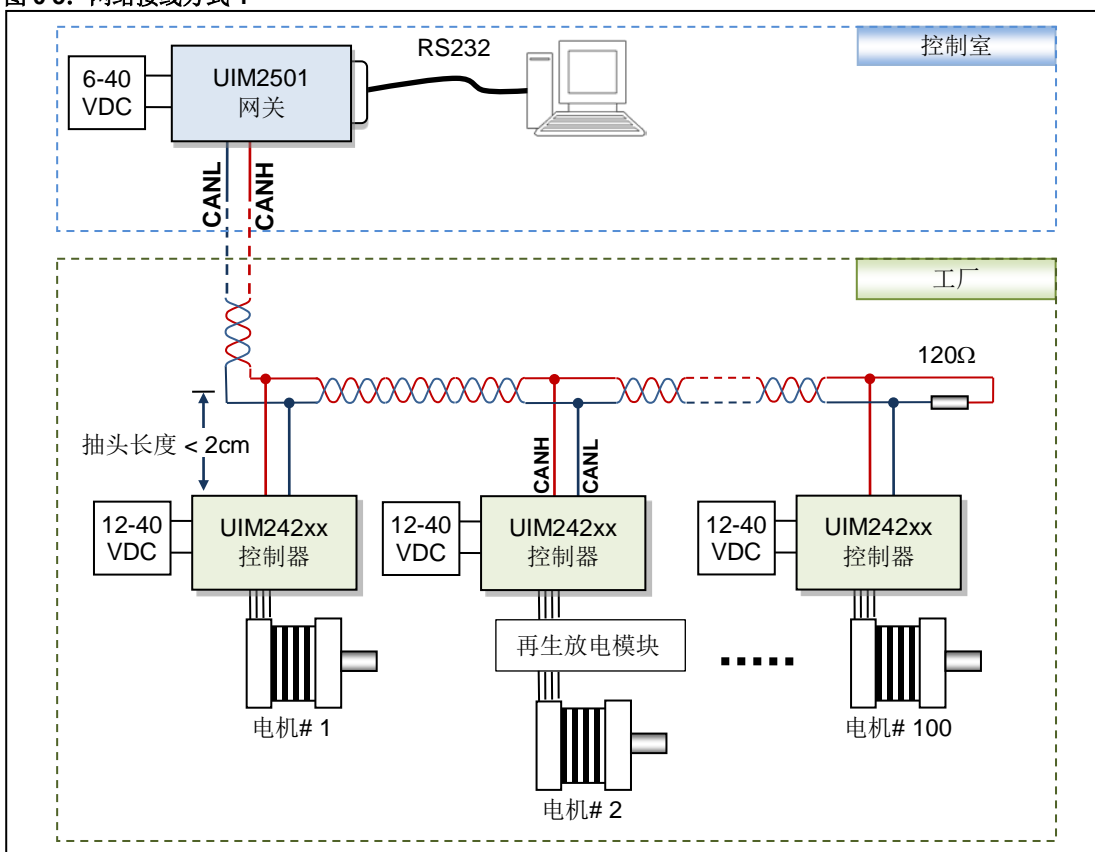
图 0-5: 网络接线方式-1
