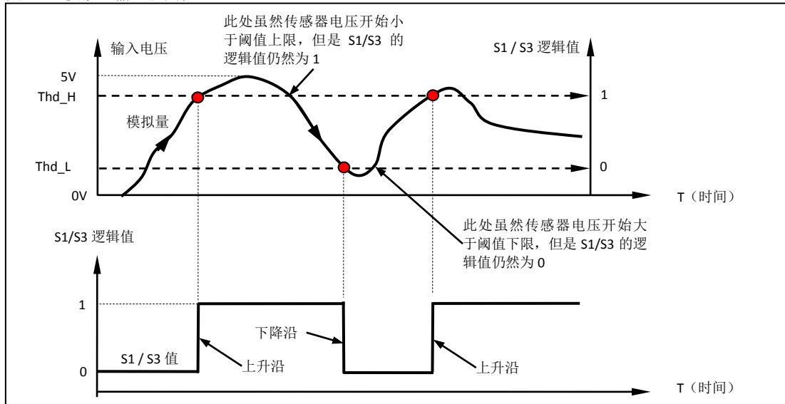
图 8-6: 模拟量输入和阈值
