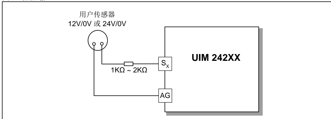
图 8-2 限流电阻
