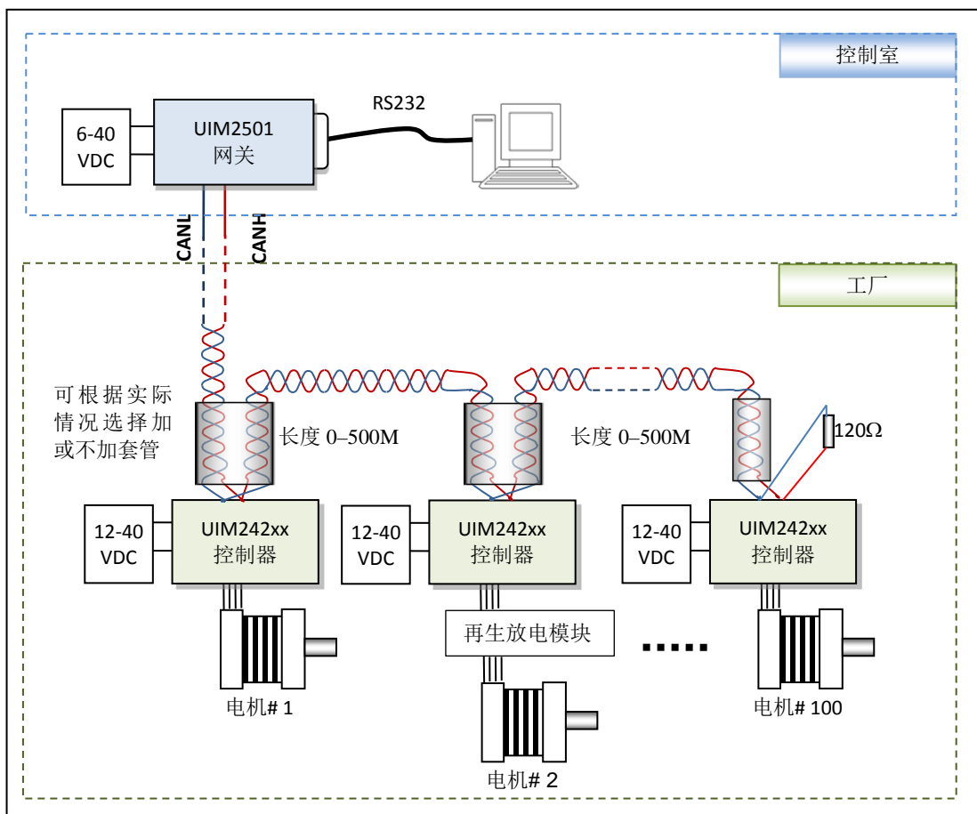
图 0-6：网络接线方式-2
